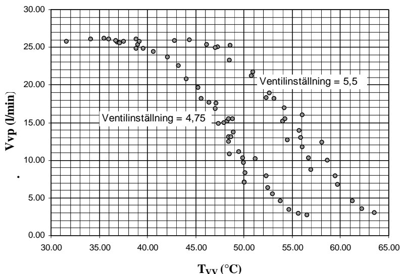
Figur 2.2. Flödet på tanksidan till tappvattenautomaten som funktion av varmvattentemperaturen för två olika ventilinställningar för Sonnenkrafts tappvattenautomat.
