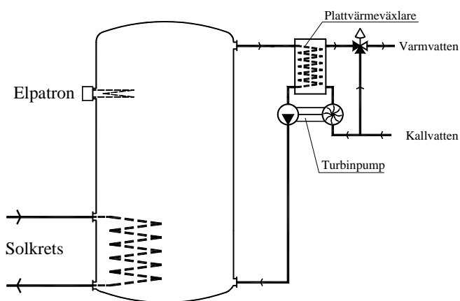
Figur 3.1. Principschema över tappvattenberedning med turbinpumpen i ett solvärmesystem med ackumulatortank
