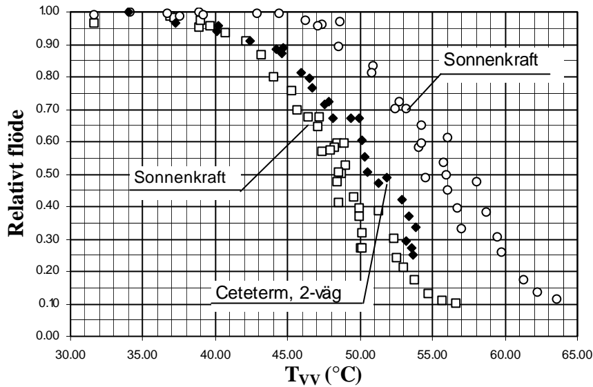
Figur 2.5. Jämförelse av reglerkaraktäristiken för Cetetherms och Sonnenkrafts tappvattenautomater. För Sonnenkraft redovisas värden för två olika ventilinställningar.
