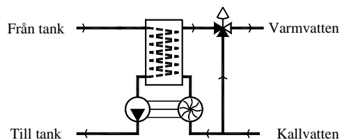
Figur 4.4. Tappvattenautomat med turbinpump och blandningsventil på varmvattensidan (Konfiguration 3A).
