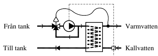
Figur 4.3. Solkraft tappvattenautomat (Konfiguration 2). Reglerutrustningen består av en flödesvakt som startar pumpen vid en varmvattentappning och en reglerventil som styr tankflödet beroende på varmvattentemperaturen. Backventilen förhindrar själv-cirkulation på tanksidan, då ingen tappning förekommer.
