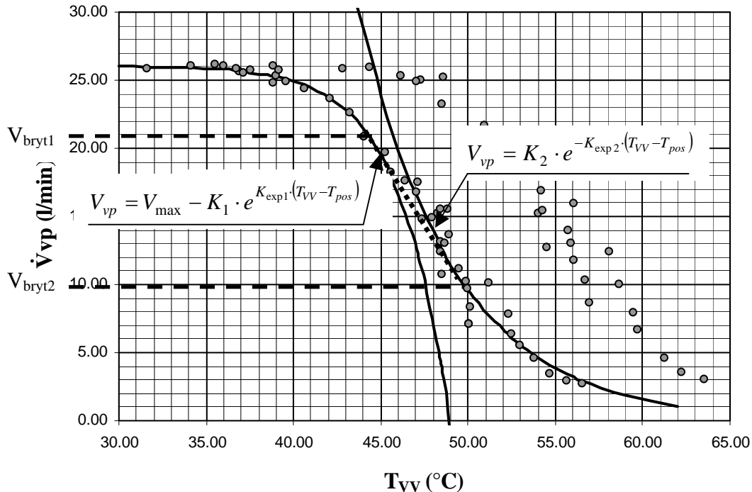
Figur 2.3. Anpassning av reglerkaraktistiken med exponentiella funktioner. Mellan V_{bryt1} och V_{bryt2} interpoleras värdena så att en linjär funktion erhålls.
