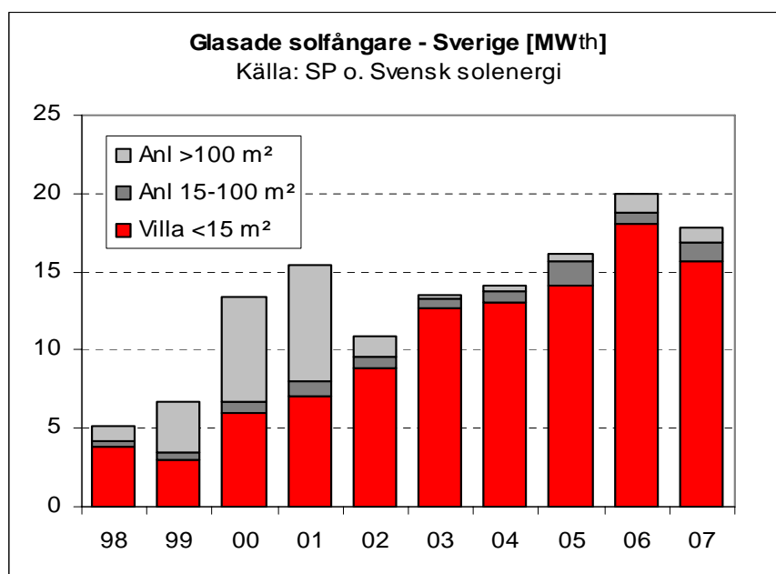
Figur 1.3. Årlig försäljning av solfångare. ( 1\text{m}^2 räknas som 0.7\text{ kW} , 20\text{ MW} motsvarar således 28\,570\text{ m}^2 ). Figuren är hämtad från referens [2] och uppdaterad med 2007.
