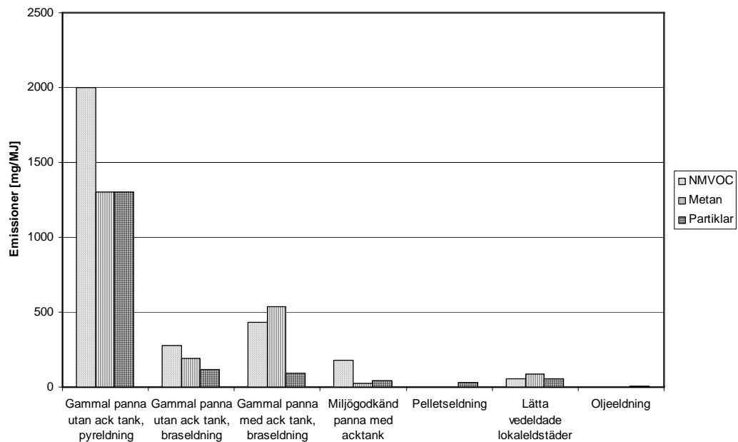
Figur 5.1. Utsläppsnivåer från olika typer av villapanor, NMVOC = lätta kolväten i rökgasen förutom metan [20].
