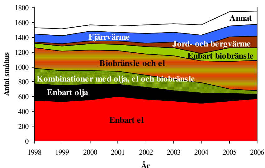
Figur 3.5. Använda energislager för permanentbebodda småhus [4, 7, 11-16] Permanentbebodda fritidshus ingår i underlaget från 2000 och jordbruksfastigheter ingår från 2005.
