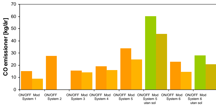
Figur 5.2. Simulerade CO-emissioner för åtta olika pelletsystem varav två varianter utan solvärme (gröna staplar). Två olika styrprinciper simuleras: On/Off-reglering och modulerande (för alla system utom System 2). Värmebehovet är cirka 15 MWh/år [31].
