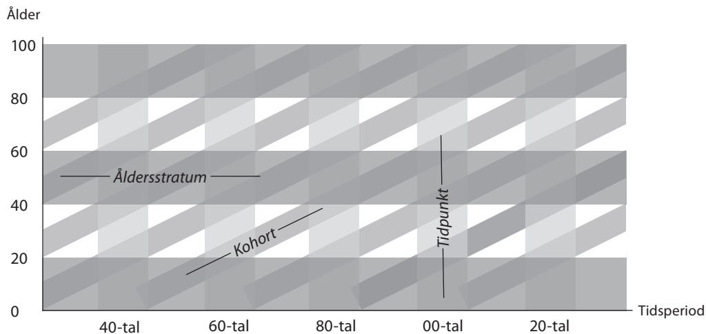
Figur 1. Kohortflödesmodell
